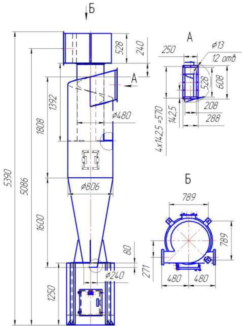
Рис.1 – Общий вид циклона ЦН 15-800 и его размеры.
